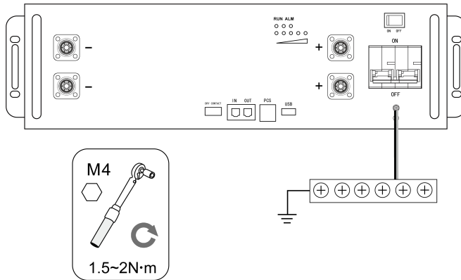
Abbildung 5-1: Installieren Sie das Erdkabel.
