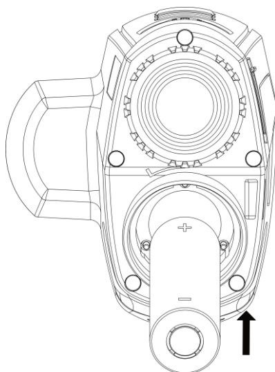
Рис. 2-2. Установка батареи
