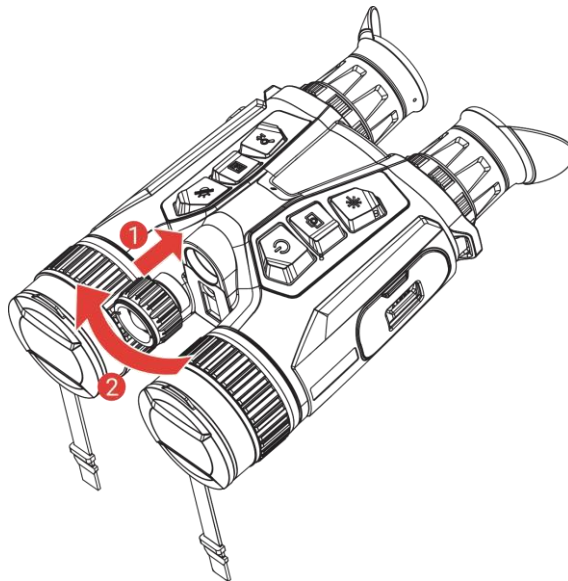
Рисунок 2-8 Установлення освітлювача
