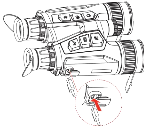
Рисунок 2-5 Заряджання пристрою
