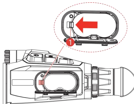
Рисунок 2-4 Виймання батареї
