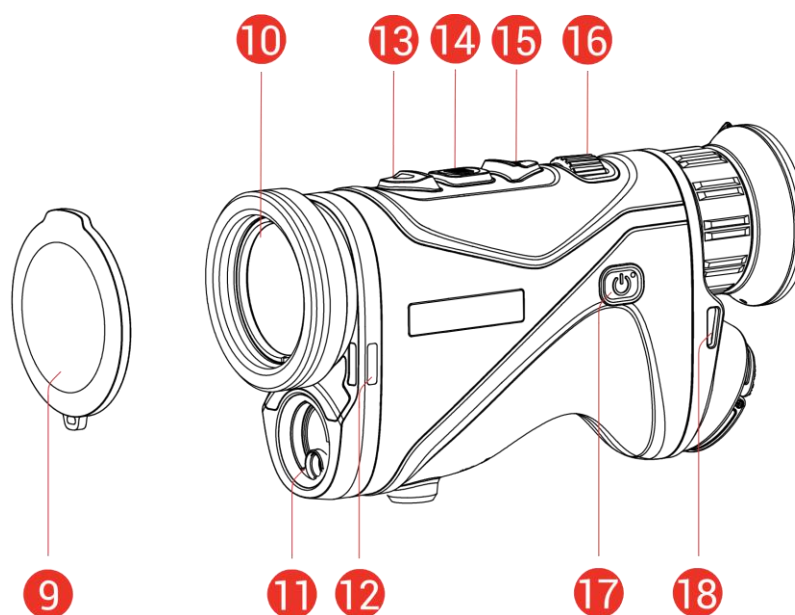
Рисунок 1-1 Зовнішній вигляд
