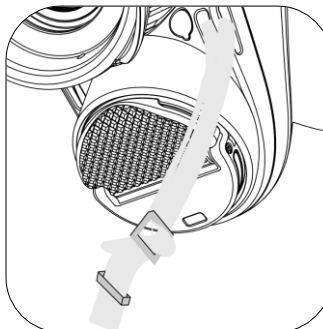
Рисунок 2-6 Протягування шийного ремінця через пряжку
