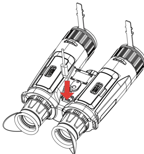
Рисунок 2-4 Підключення кабелю
