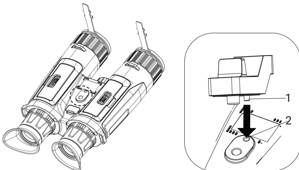
Рисунок 2-8 Розташування та вставлення перехідника
